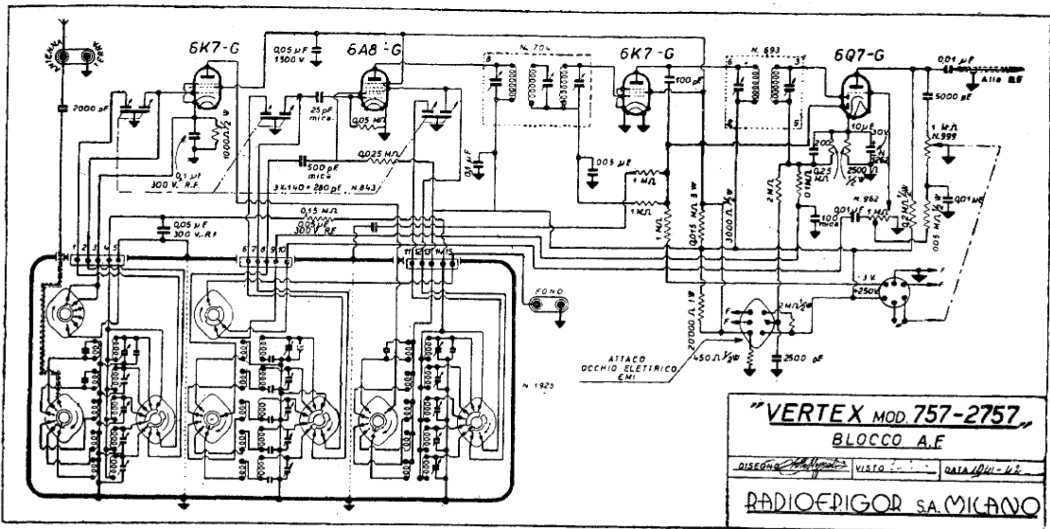
VERTEX (S. A. RADIO FRIGOR). — Mod.757 e 2757. — Produzione 1941-1942. — Media frequenza: 467 kHz. Avvolgimento di campo: 1200 ohm. — Per la parte alimentatrice e amplificatrice finale v. lo schema seguente.
